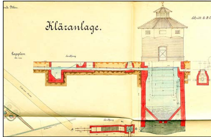
Projektzeichnung des Klärwerkes für Dölau, das nach 1896 gebaut werden sollte, aber durch den 1. Weltkrieg nie entstand. Repro: Dr. Wissenbach
